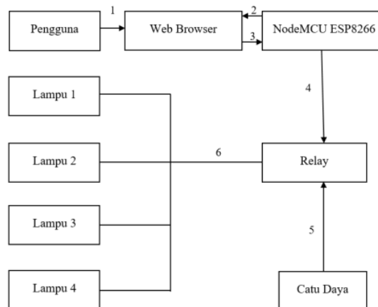
Gambar 2 Blok Diagram Sistem Secara Keseluruhan
