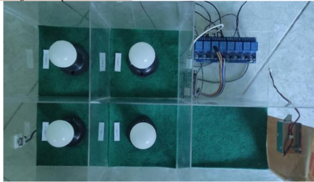
Gambar 5 Perancangan Alat Secara Keseluruhan
