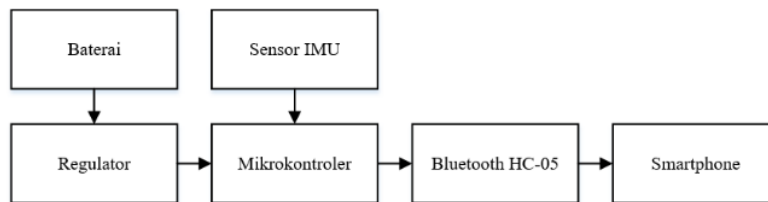
Gambar 4. Blok Diagram Sistem Secara Keseluruhan
